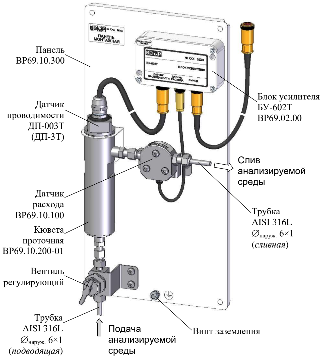
Рисунок 2.10 – Расположение датчика проводимости ДП-003Т (ДП-3Т) на панели монтажной VP69.10.000 (проточный способ измерений)
