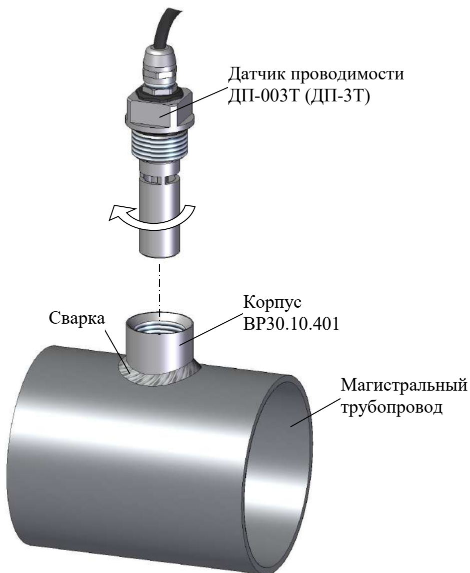
Рисунок 2.12 – Установка датчика проводимости ДП-003Т (ДП-3Т) в магистральный трубопровод
